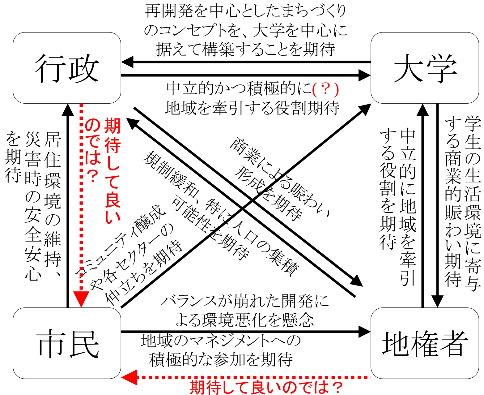
図. 再開発の主要なステークホルダー相互の期待
