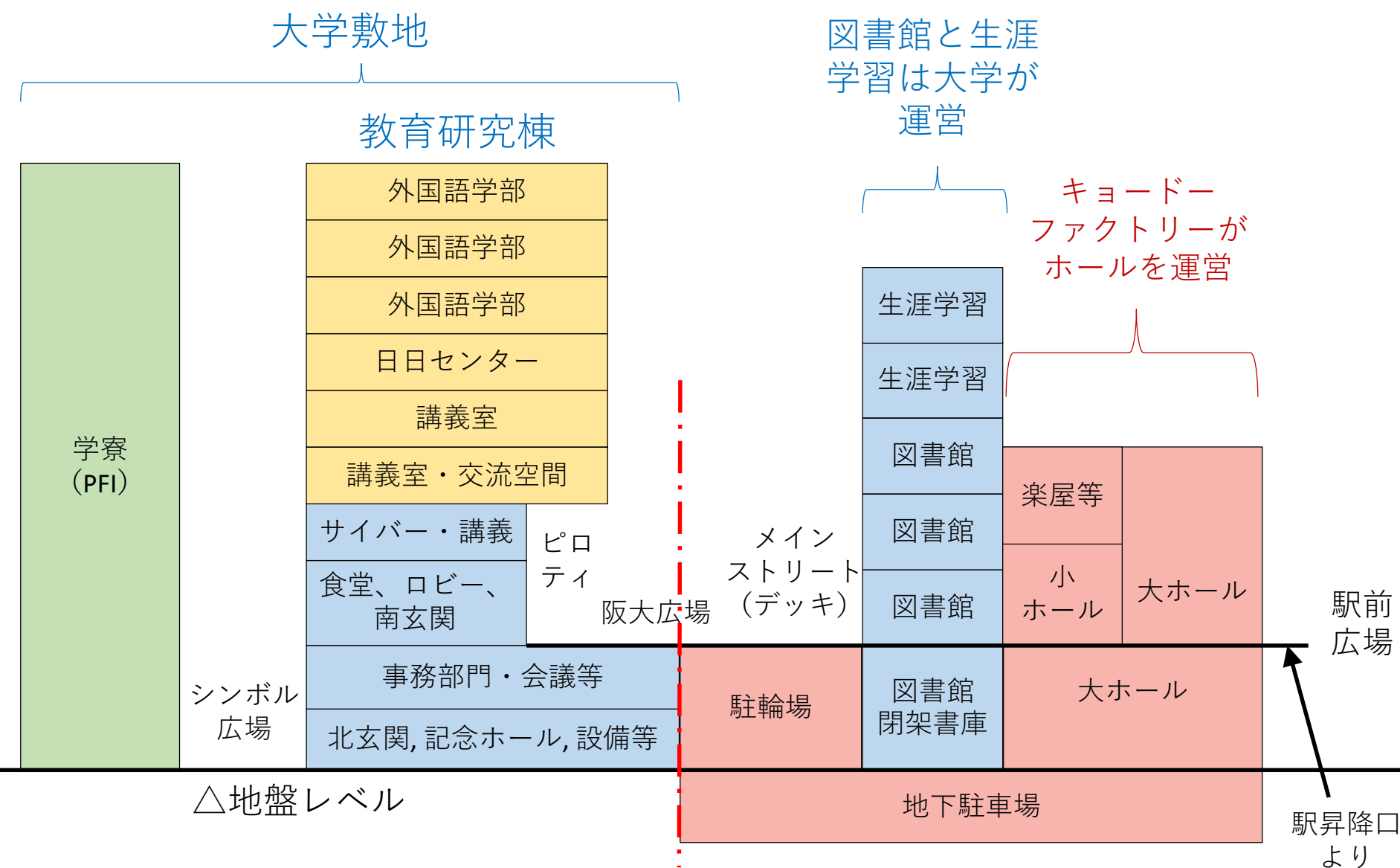
模式断面図 Model Section
